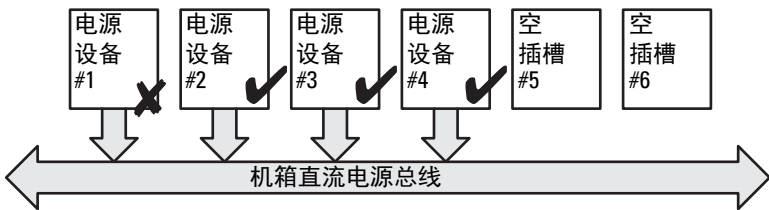
图 9-2. 电源设备冗余：合计 4 个 PSU，其中 1 个 PSU 故障。
