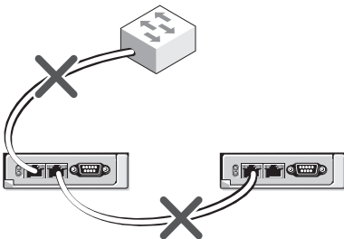
图 2-4. CMC 网络连接布线错误 - 2 个 CMC
