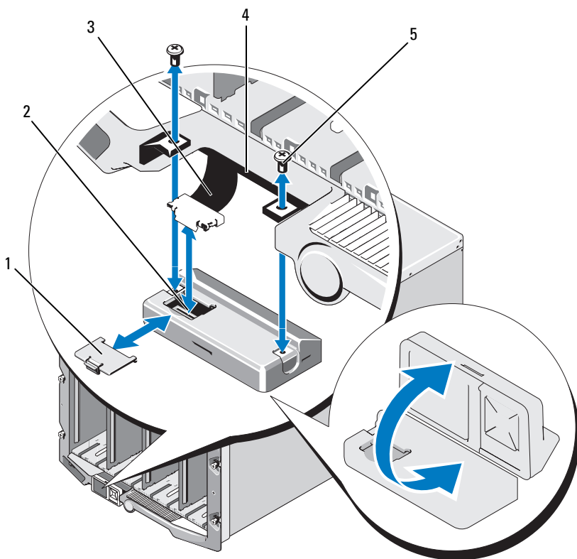
图 13-1. 卸下和安装 LCD 模块
