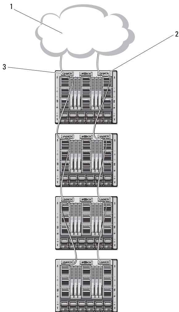
图 2-1. 菊花链式 CMC 网络连接
