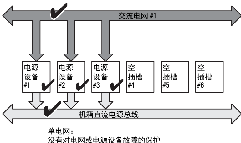
图 9-3. 机箱中 3 个 PSU 且无冗余
