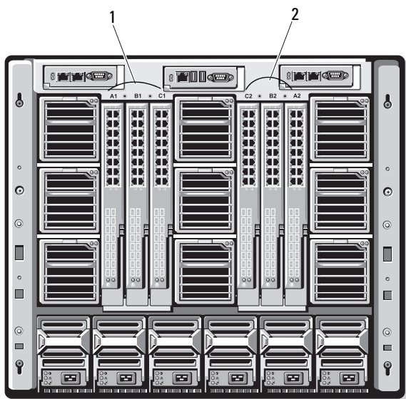
图 11-1. 机箱后视图，显示 IOM 的位置
