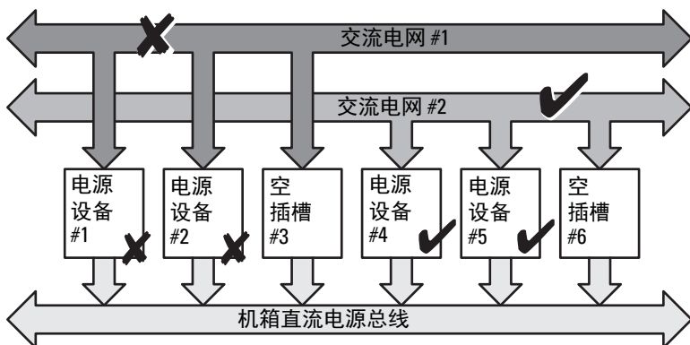
图 9-1. 每个电网 2 个 PSU 和电网 1 上的供电故障
