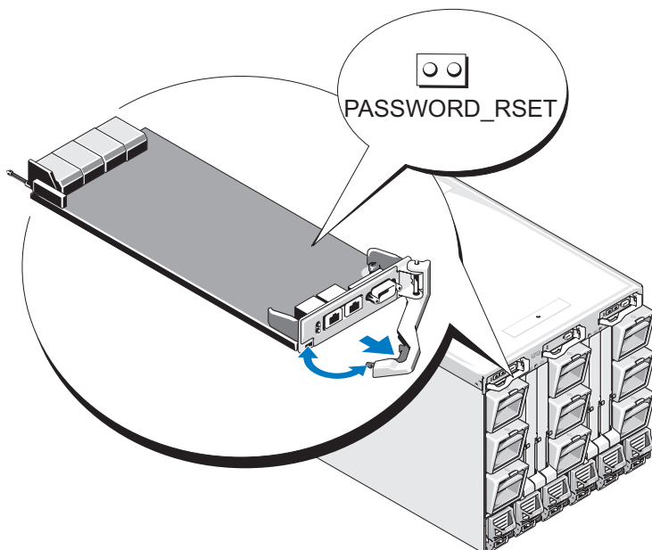
图 12-1. 密码重设跳线位置
